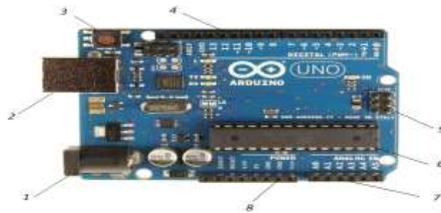
1-rasm. Arduino Uno qurilmasi tuzilish tasnifi.
